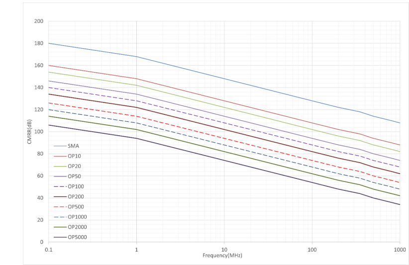
衰减器 CMRR 曲线：上图展示不同型号衰减器（0dB）在各个频率下的共模抑制能力。
