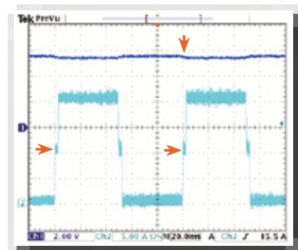
图 4：并联非同步动态负载
