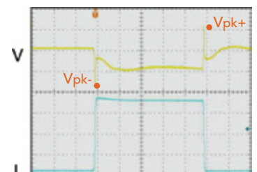
图 2：电压峰值量测
