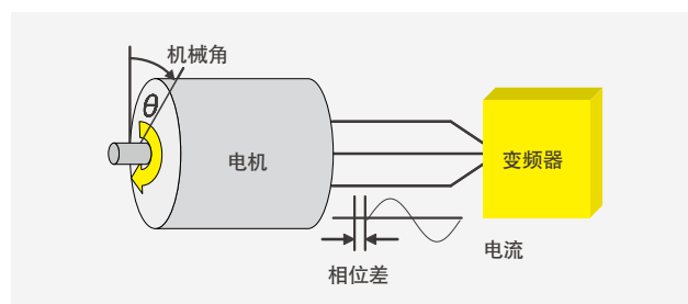
电角度测量示例
